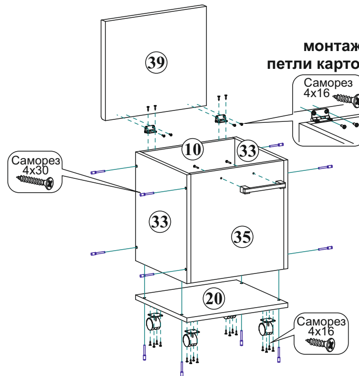
Схема выкатной тумбы
