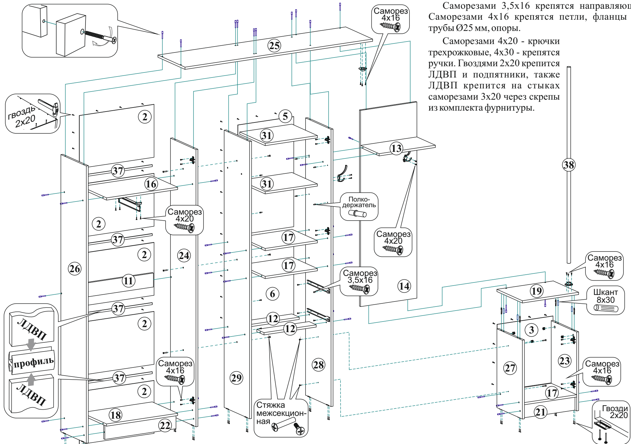
Секция «тумба», «шкаф с ящиками», «шкаф» фиксируются между собой межсекционными стяжками. Предварительно, под них необходимо просверлить отверстия Ø 5мм.
